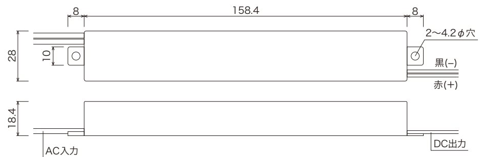
製品図面
