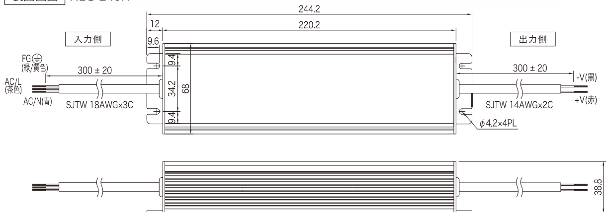
製品図面 HLG-240H
